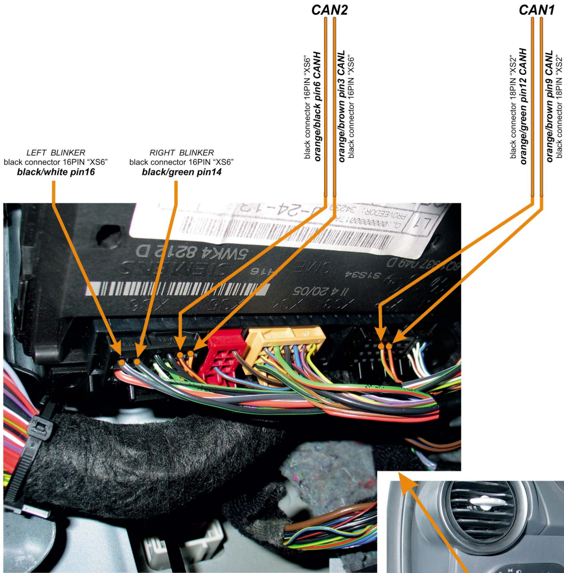
CONTROLLER MODULE
